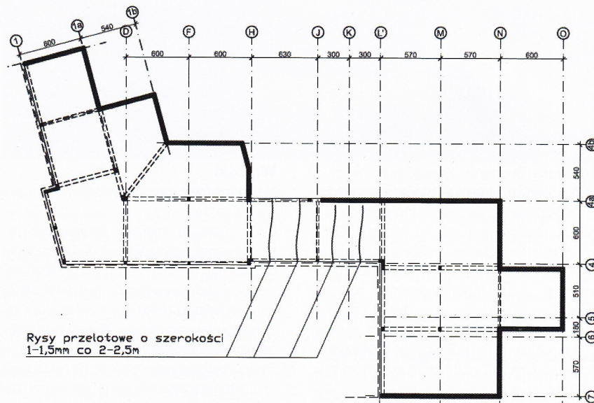
Rys. 2. Schemat analizowanego fragmentu stropu
