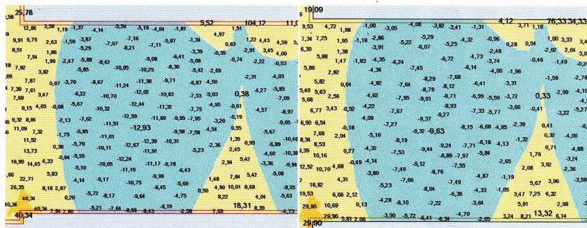
Rys. 5. Momenty zginające w płycie w kierunku prostopadłym do rys przy obciążeniu użytkowym p=3,0 \text{ kN/m}^2 :
