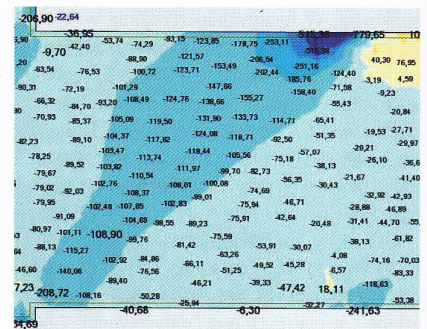
Rys. 6. Siły rozciągające (kierunek y-y) przy obciążeniu temperaturą -15^\circ\text{C}
