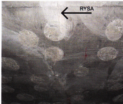
Rys. 3. Rysy w konstrukcji
