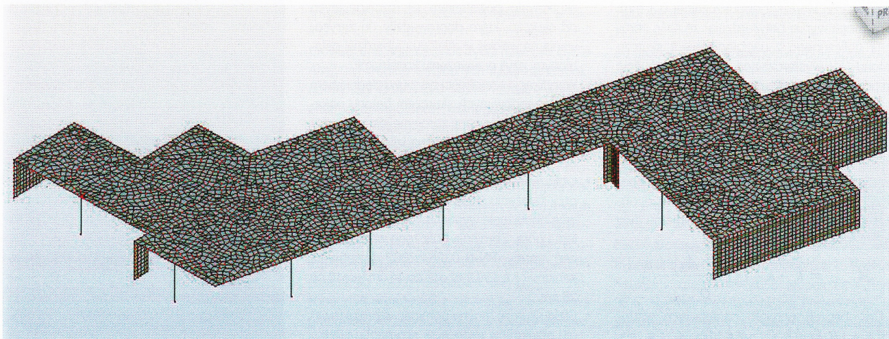
Rys. 4. Model obliczeniowy płyty w systemie MES
