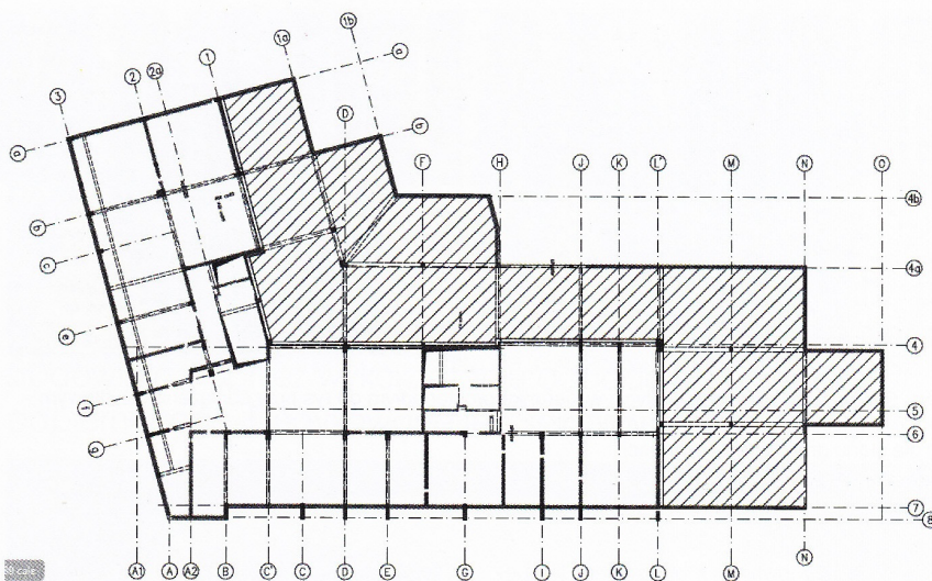
Rys. 1. Rzut budynku w kondygnacji garażu
